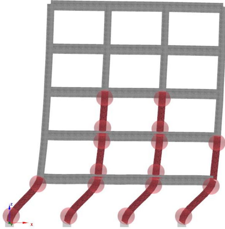
Görsel 5. Referans bina modeli için kesme kuvvet hasar durumu ve oluşan plastik mafsallar
