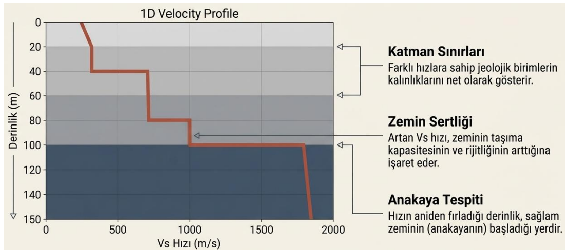
Görsel 7. Örnek bir V_s hız modeli
