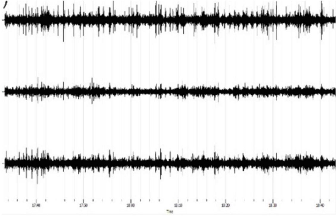
Görsel 1. Üç bileşenli bir mikrotremor kaydı.
