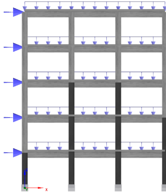
Görsel 6. Güçlendirilen kolonlar için elde edilen iki boyutlu model
