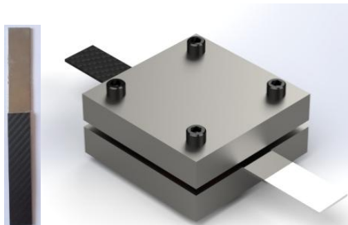
Görsel 2. TBB bağlantısı ve yapıştırma bağlantı kalıbı
