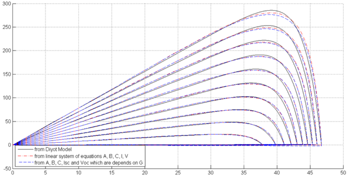
Görsel 3. Matlab Programı Kullanılarak Akbaba Modeli İçin P-V Karakteristikleri.
