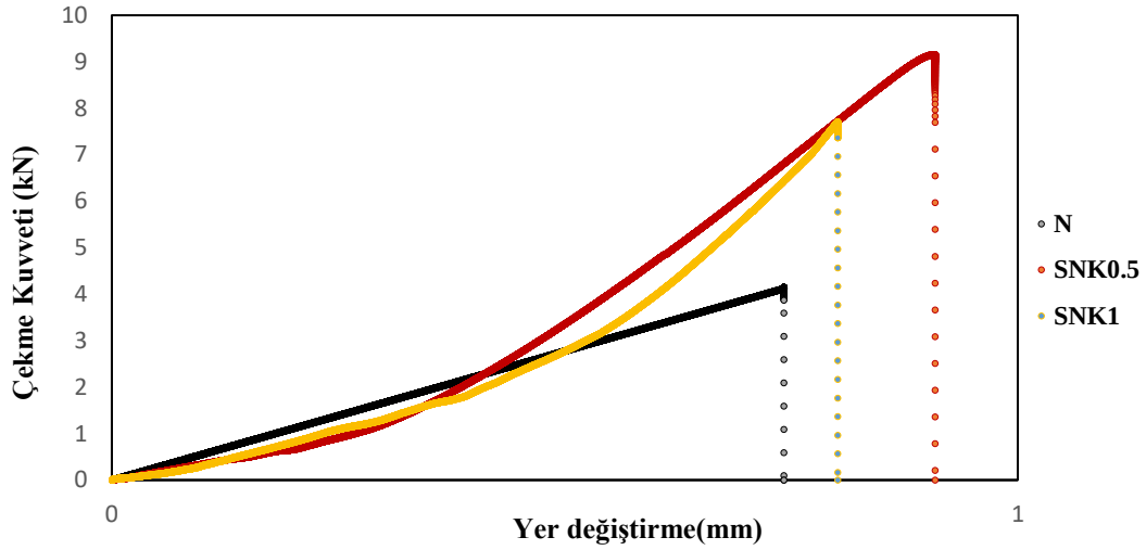
Görsel 3. Farklı nano SNK konsantrasyonlarına sahip TBB numunelerinin çekme kuvveti-yerdeğıştirme grafikleri
