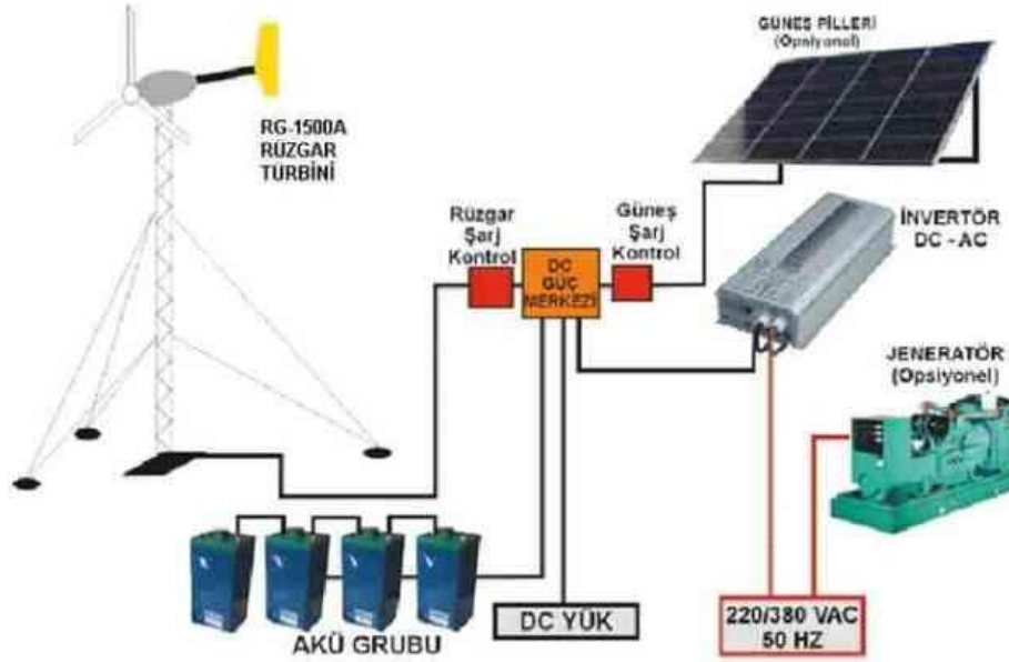
Figure 1. Hibrit Enerji Sistemlerinde Kullanılan Cihazlar ve Düzenlemeleri [14]
