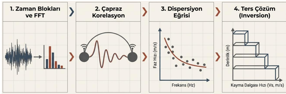
Görsel 6. SPAC yöntemi veri işlem adımları
