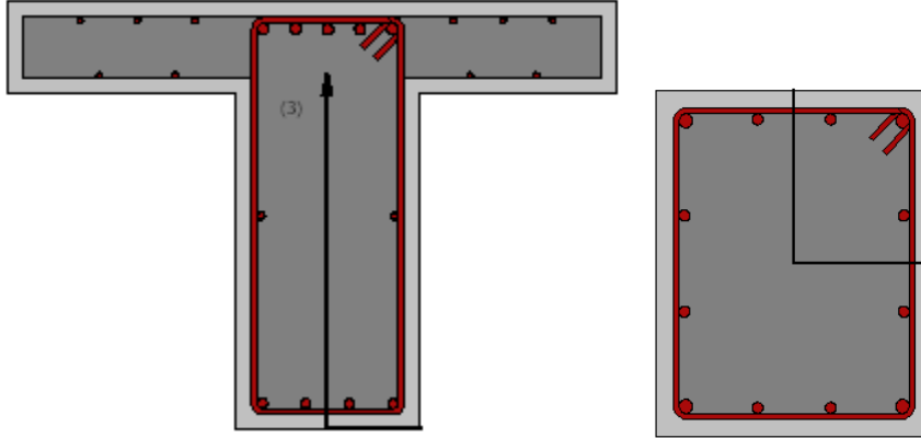
Görsel 2. Dikkate alınan kiriş ve kolon en kesitleri
