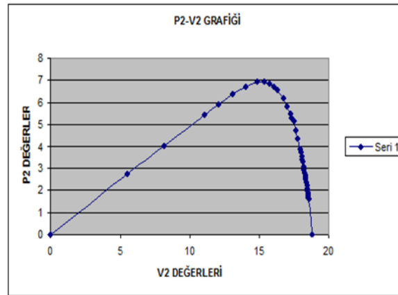
Görsel 2. P-V Karakteristik eğrisi Işınım %50
