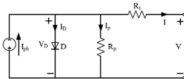
Görsel 1. Fotovoltaik Hücresinin Tek Diyotlu Elektrik Eşdeğer Modeli.
