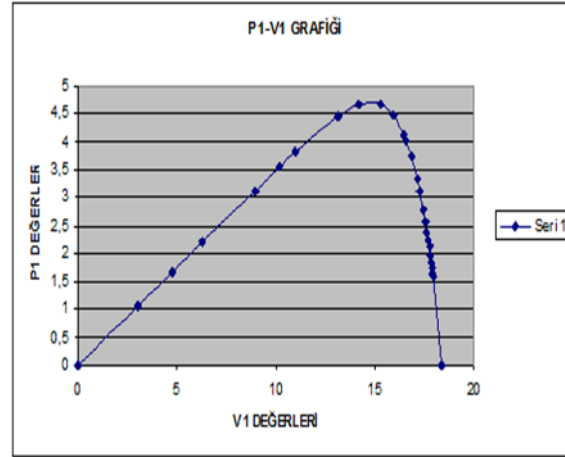
Görsel 1. P-V Karakteristik Eğrisi Işınım %35
