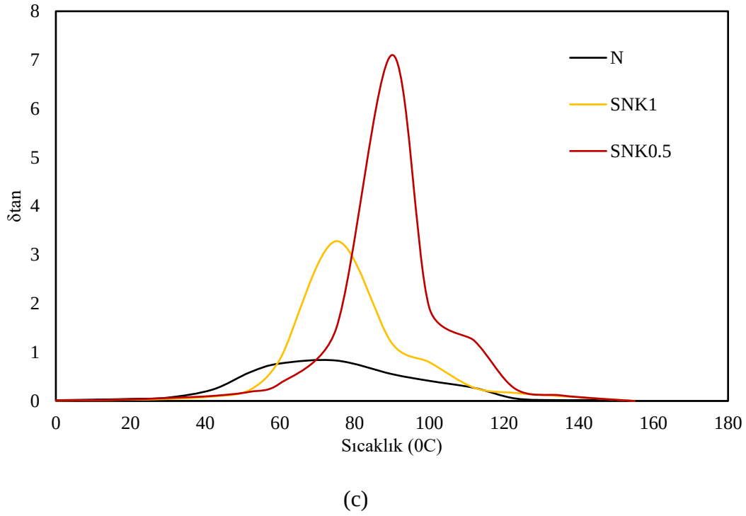
Görsel 4. Nano-modifiye yapıştırıcıların sıcaklığa bağlı: (a) Depolama modülü, (b) Kayıp modülü ve (c) Tan delta değişimleri
