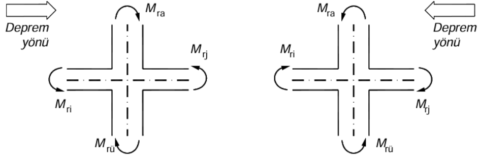
Görsel 1. Kolon-kiriş birleşim noktasında oluşacak momentler (TBDY-2018)
