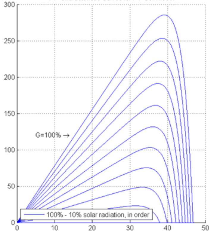
Görsel 2. Matlab Programı Kullanılarak Geleneksel Diyot Modeli İçin P-V Karakteristikleri.
