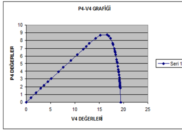
Görsel 4. P-V Karakteristik Eğrisi ışınlım %100
