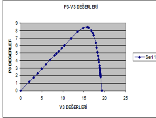
Görsel 3. P-V Karakteristik Eğrisi ışınlım %85
