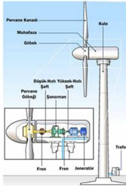
Figure 2. Rüzgar Türbininin Parçaları [15]
