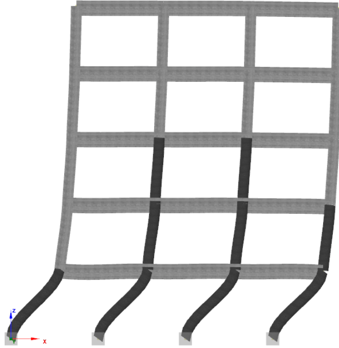
Görsel 7. Önerilen güçlendirme sonrası elde edilen kesme kuvveti için deformasyon durumu
