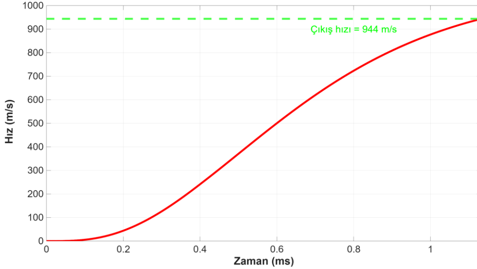
Şekil 3. Mermi hızının zamana bağlı değişimi
