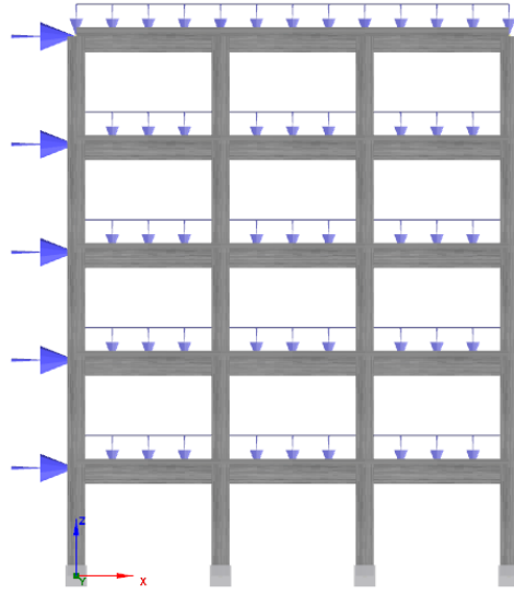
Görsel 3. Dikkate alınan 2 boyutlu model
