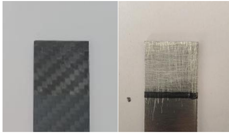
Görsel 1. Taşlanmış KFTP ve AA7075-T6 numunelerinin yüzey görüntüleri
