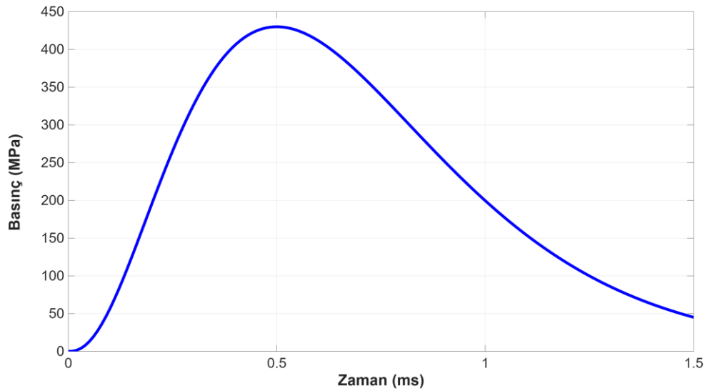
Şekil 1. Barut gazı basıncının zamana bağlı değişimi
